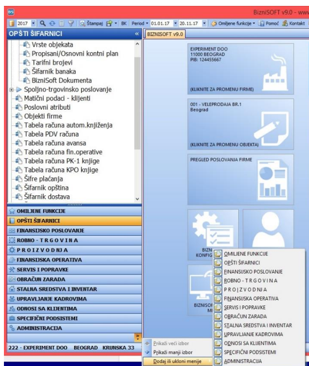
Izbor menija
