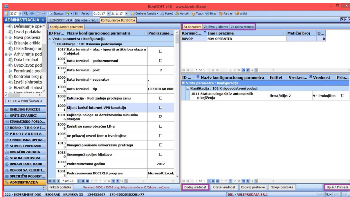
BizniSoft konfigurator
